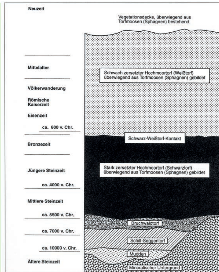
Schematische Querschnittzeichnung: Moorschichten
